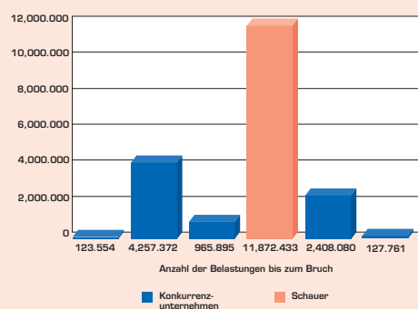
Lebensdauer des Schauer Förderseils
